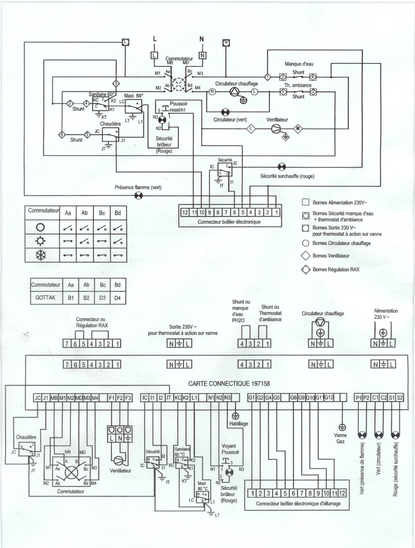
Figure 19 - Schéma et câblage électrique
