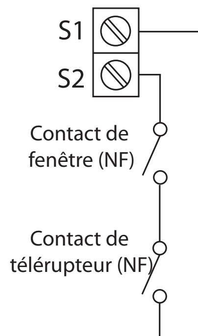
Configuration pour contact de fenêtre ou d'autres contacts comme un télerupteur
