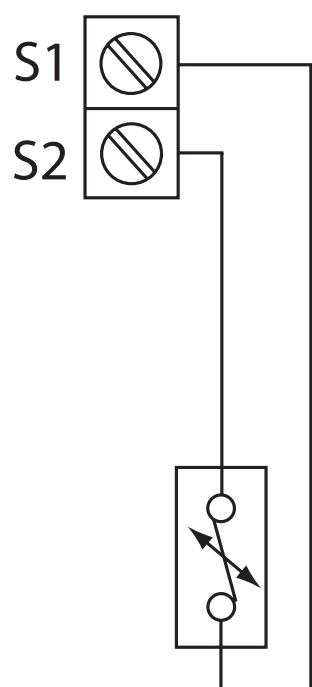
Configuration pour capteur d'ambiance à distance ou pour capteur de limite
