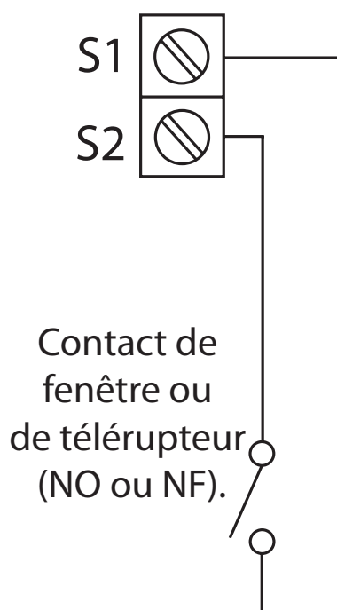
Configuration pour contact de fenêtre ou autre contact comme un télerupteur.
